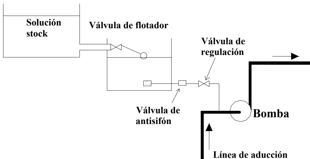
Dosificador en tubería de aducción
