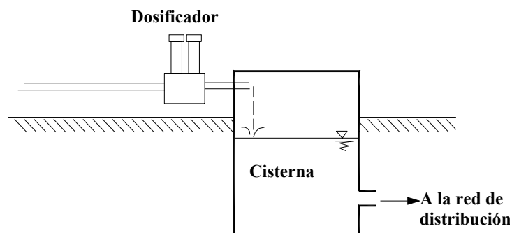
Instalación típica de un clorador por erosión de Tablet de hipoclorito de calcio
