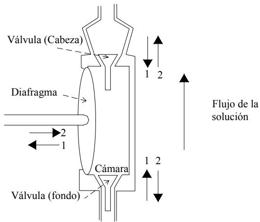
Detalle operativo del cabezal con su diafragma
