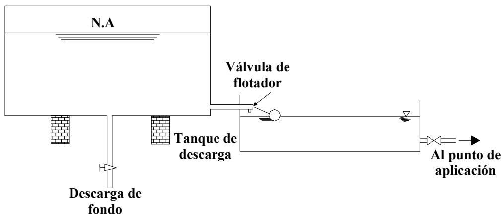
Tanque con válvula de flotador
