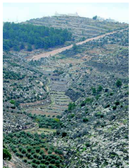
Warping dams, Palestine. (N. Harari)
