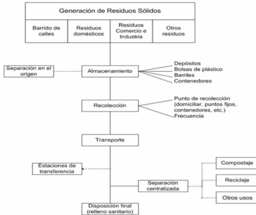
Figura 2.2 Elementos físicos del sistema de manejo de residuos sólidos.
