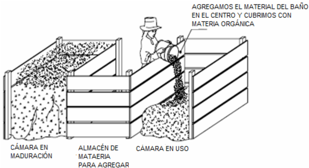
Figura 4.16 Cámaras de tratamiento exteriores.
