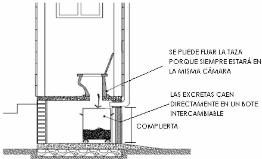
Figura 3.9 Arreglo para un baño con composteo exterior.
