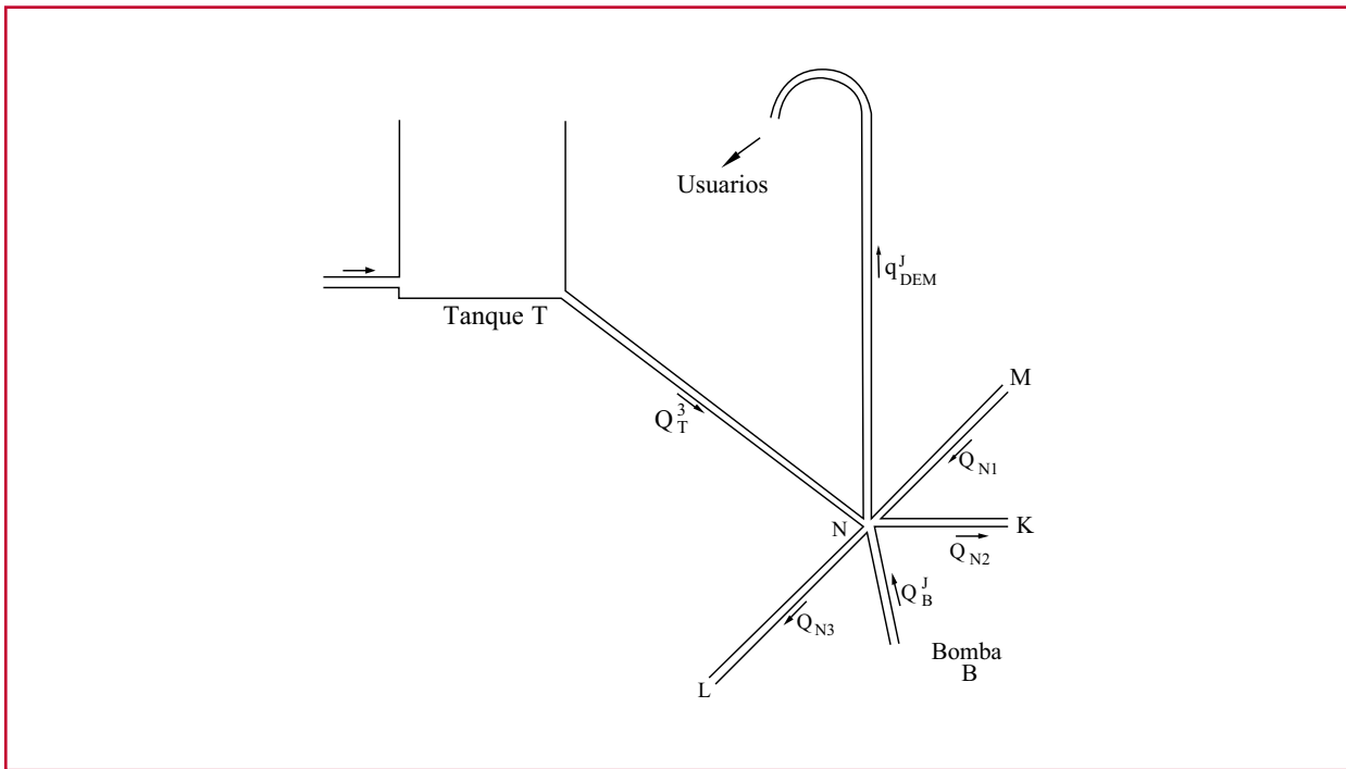
Ilustración 3.14 Nodo N de la red
