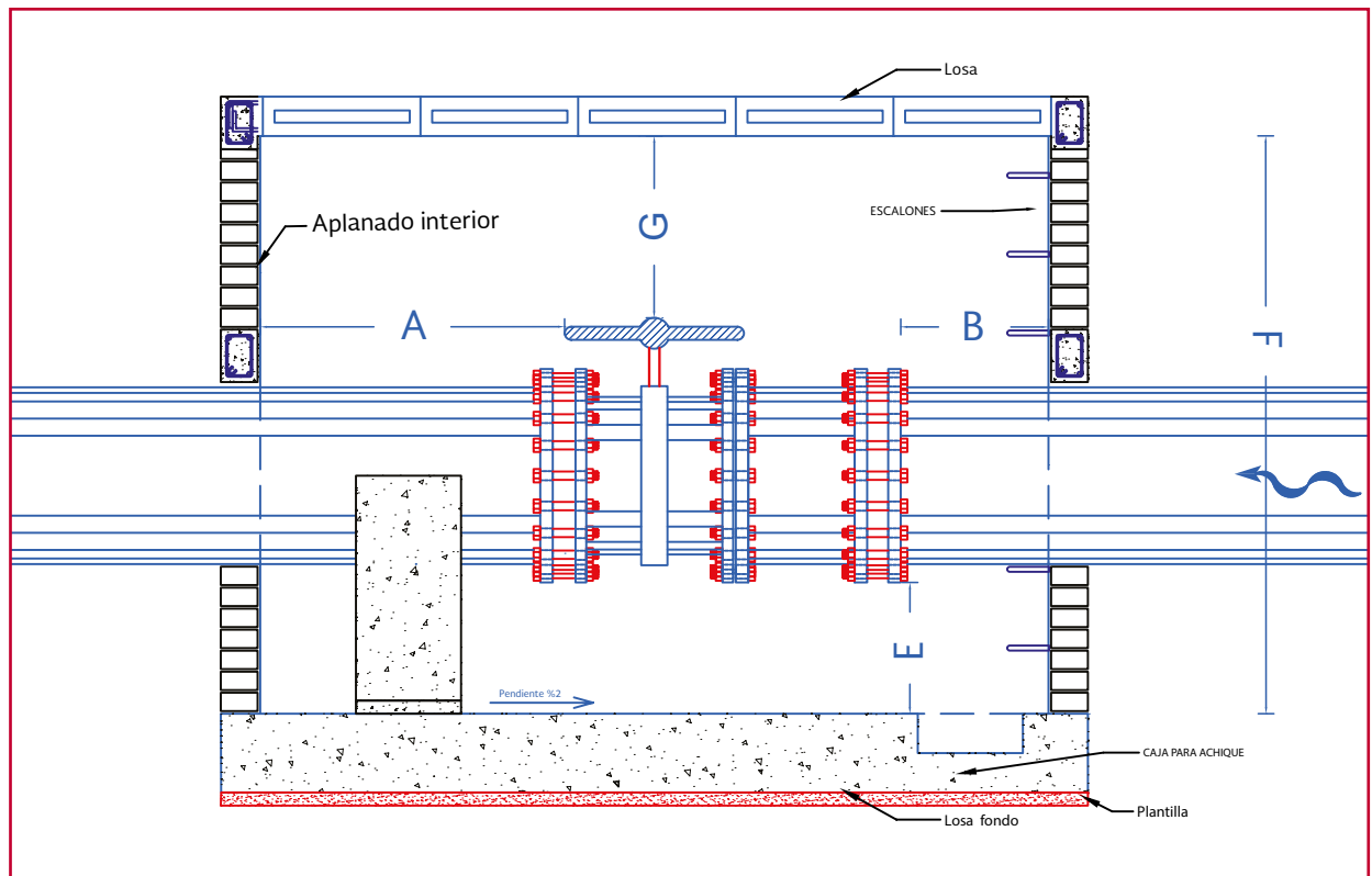
Ilustración 2.18 Caja de válvula (Elevación)
