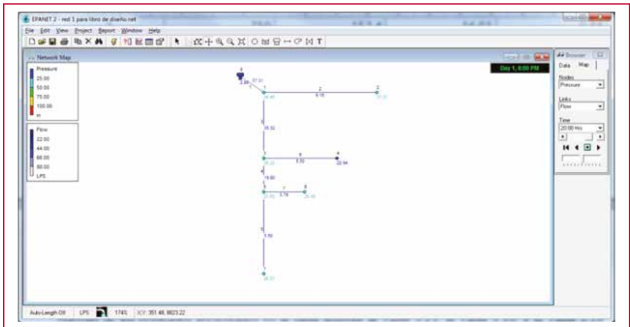
Ilustración 3.17 Simulación en los nodos del funcionamiento hidráulico de la red a las 20:00 h
