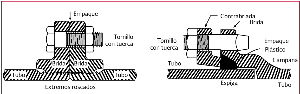
Ilustración 2.5 Unión bridada y unión mecánica
