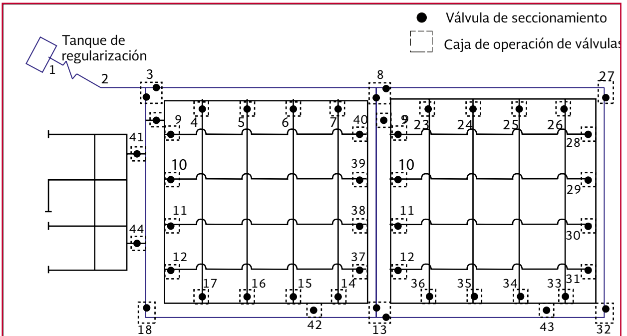
Ilustración 1.5 Red secundaria en bloques y en dos planos
