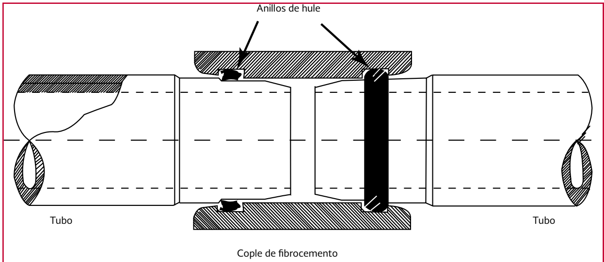
Ilustración 2.3 Unión por medio de coples de fibrocemento
