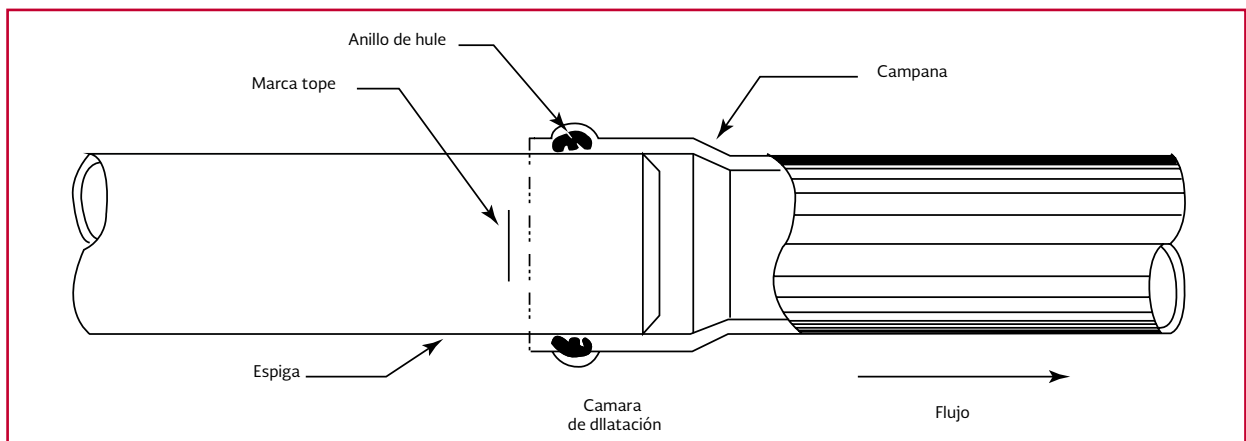
Ilustración 2.1 Unión espiga-campana en tubería de PVC
