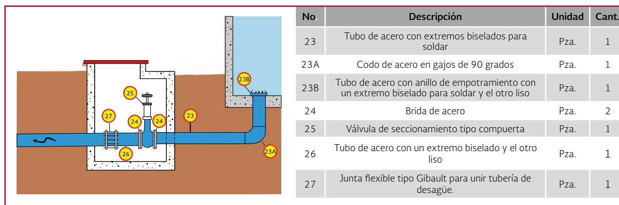
Ilustración 2.39 Fontanería de salida con desagüe de fondo
