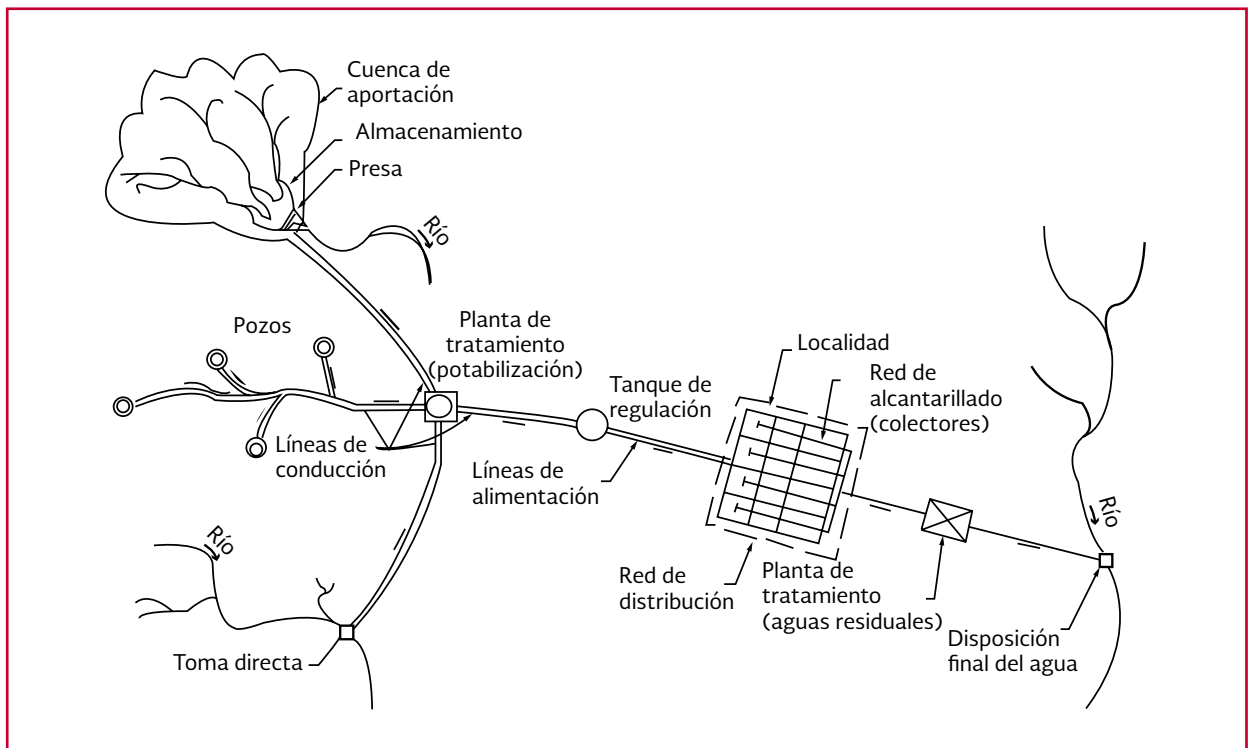
Ilustración 1.1 Configuración típica de un sistema de abastecimiento de agua en localidades urbanas
