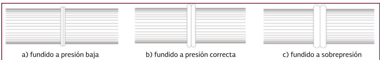
Ilustración 2.2 Unión por termo fusión
