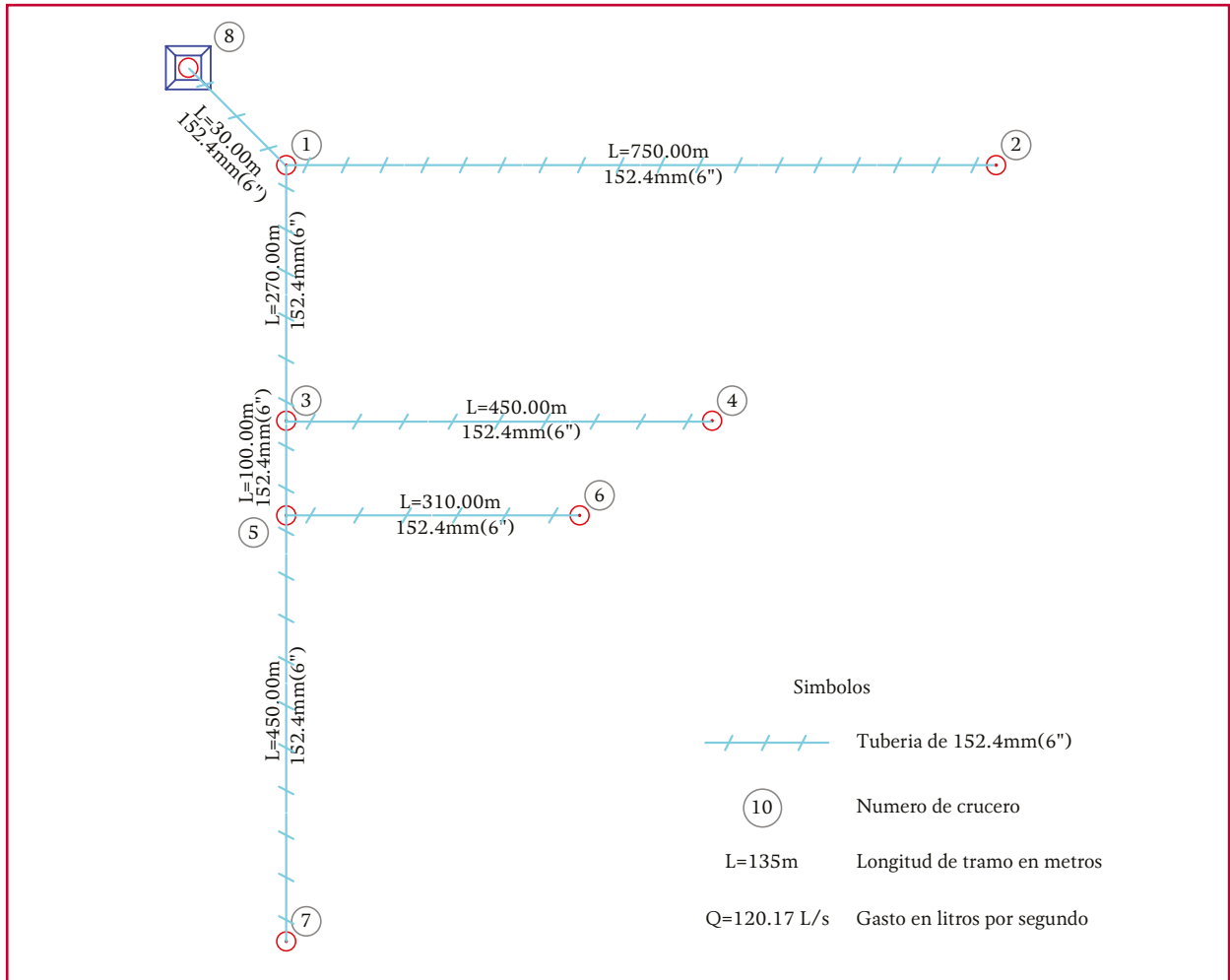
Ilustración 3.4 Red abierta de agua potable para el ejemplo
