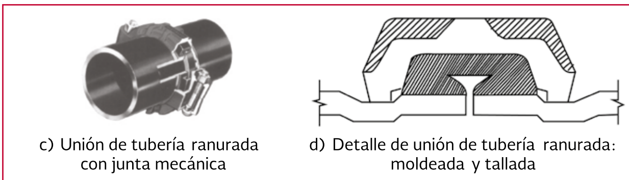
Ilustración 2.10 Uniones para tubería de acero
