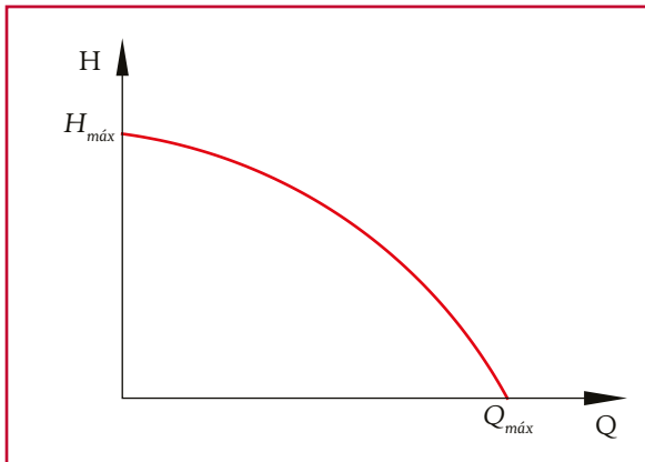
Ilustración 3.13 Curva característica carga-gasto de la bomba
