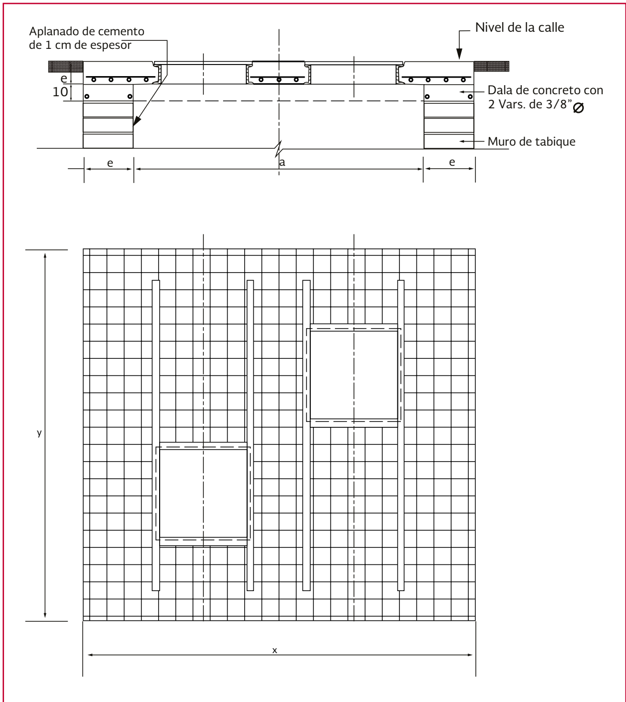
Ilustración 2.33 Caja tipo 11
