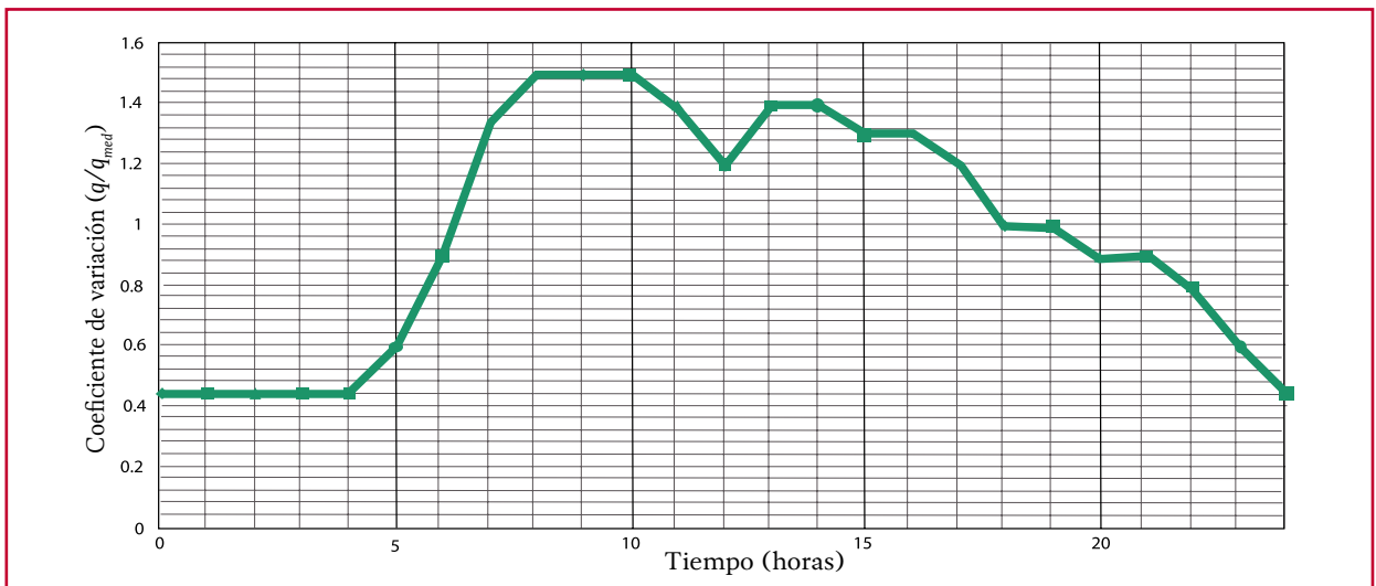
Ilustración 3.11 Coeficientes de variación horaria para pequeñas comunidades
