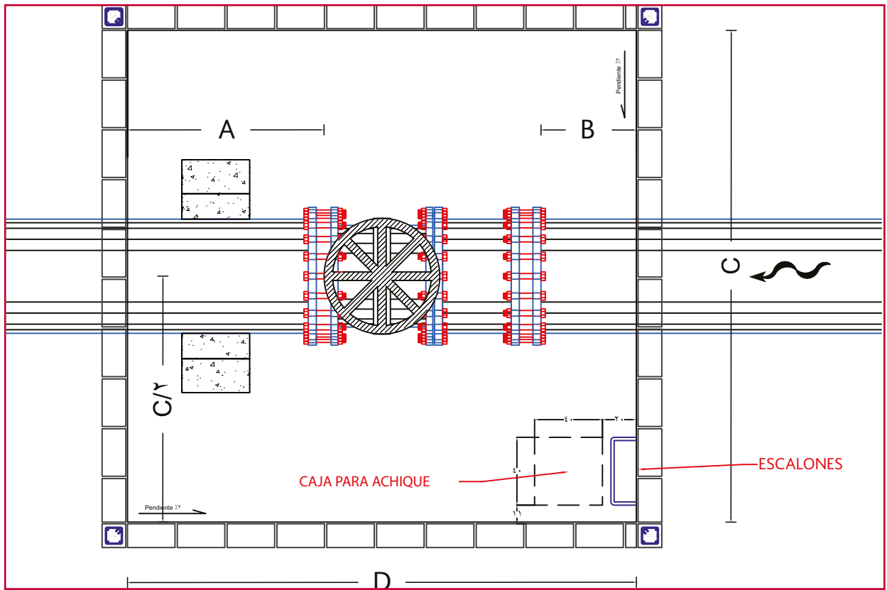
Ilustración 2.17 Caja de válvula (Planta)
