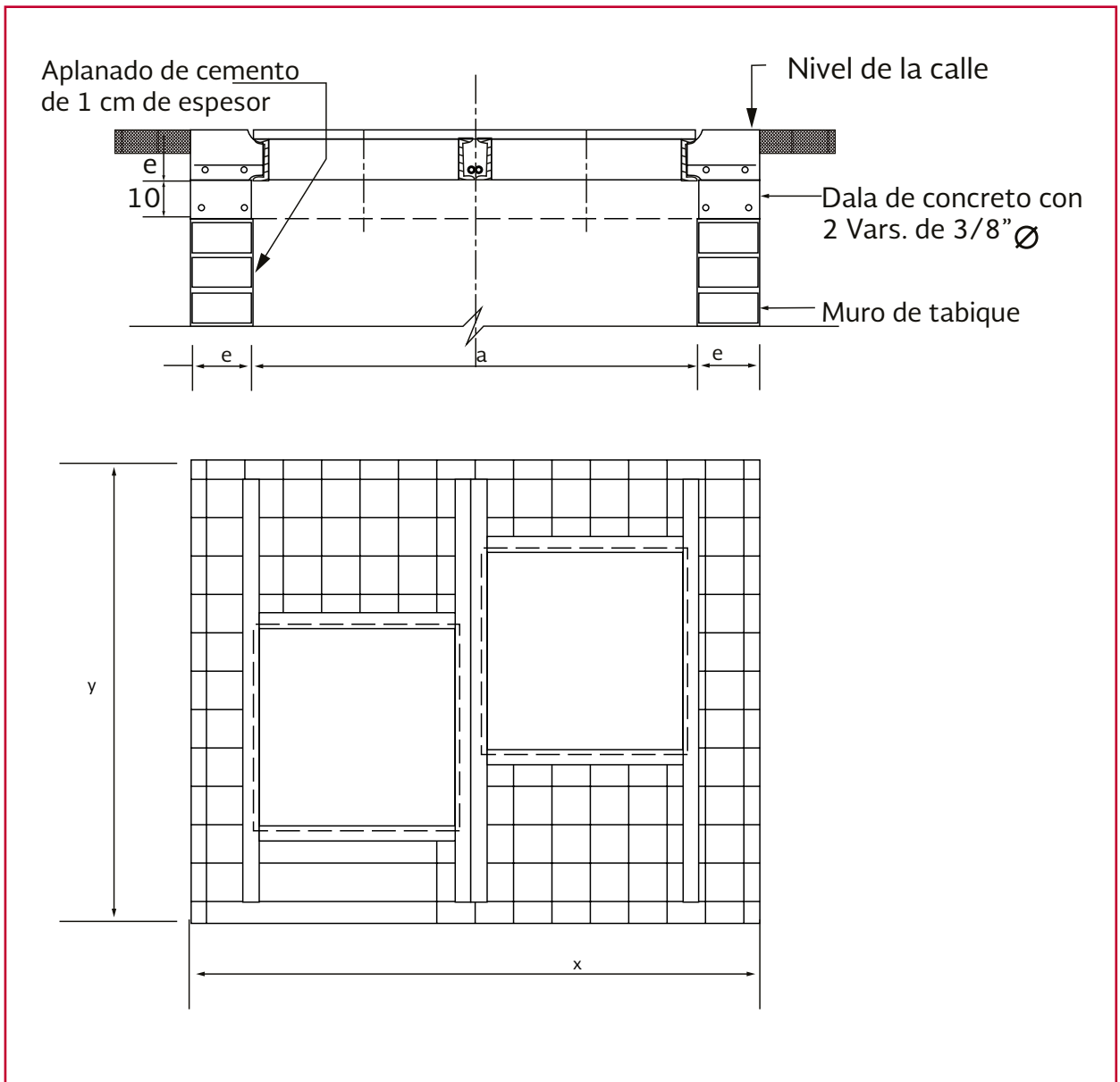
Ilustración 2.31 Caja tipo 9
