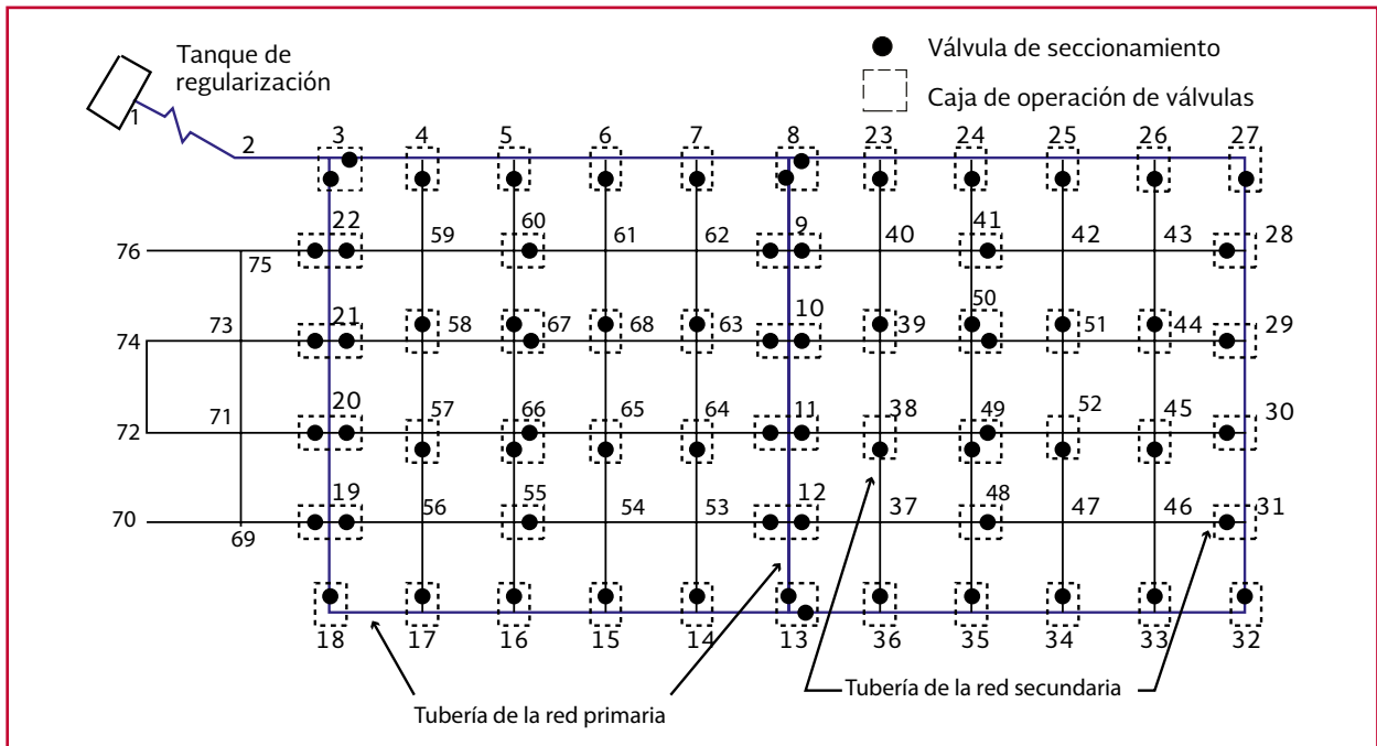
Ilustración 1.2 Red secundaria convencional
