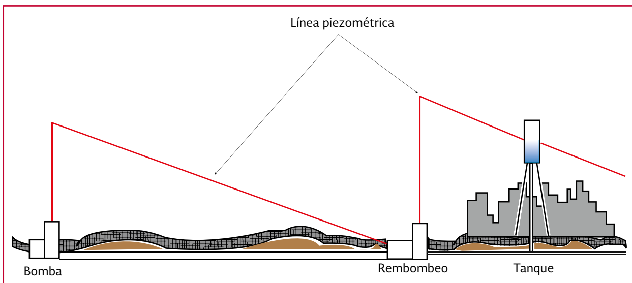
Ilustración 1.7 Distribución mixta (no recomendable)
