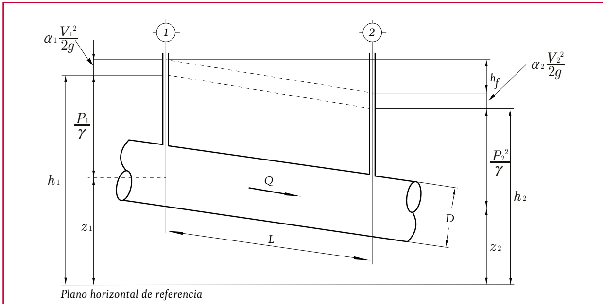
Ilustración 3.1 Cargas en los extremos del tubo
