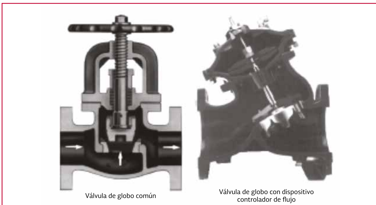
Ilustración 2.15 Válvulas de globo
