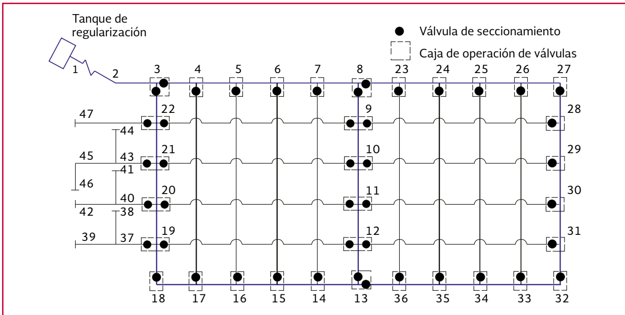
Ilustración 1.3 Red secundaria en dos planos
