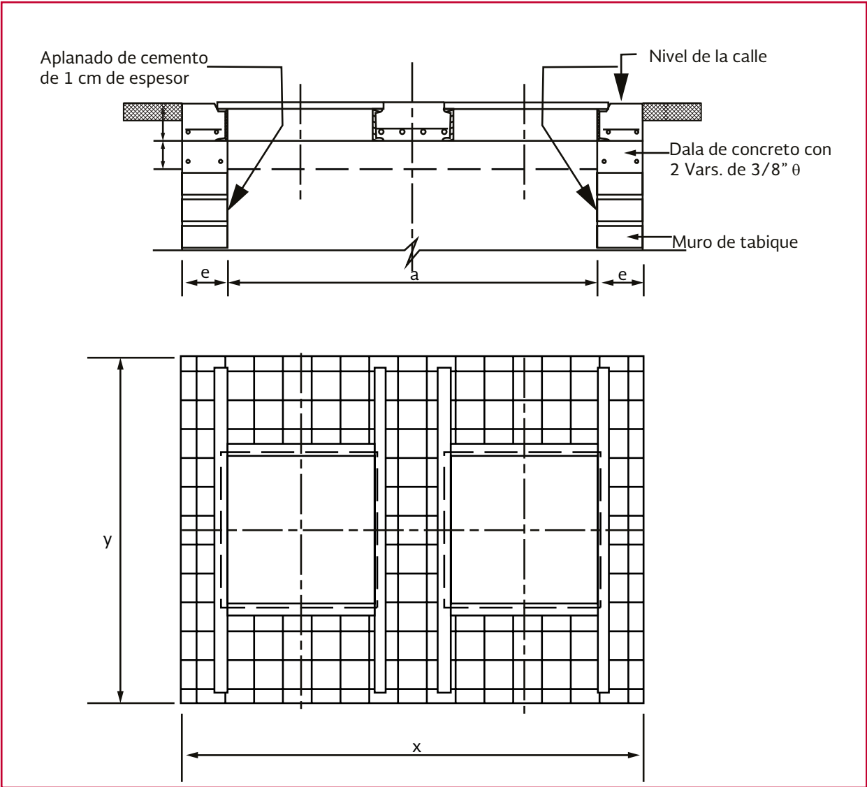
Ilustración 2.27 Caja tipo 5
