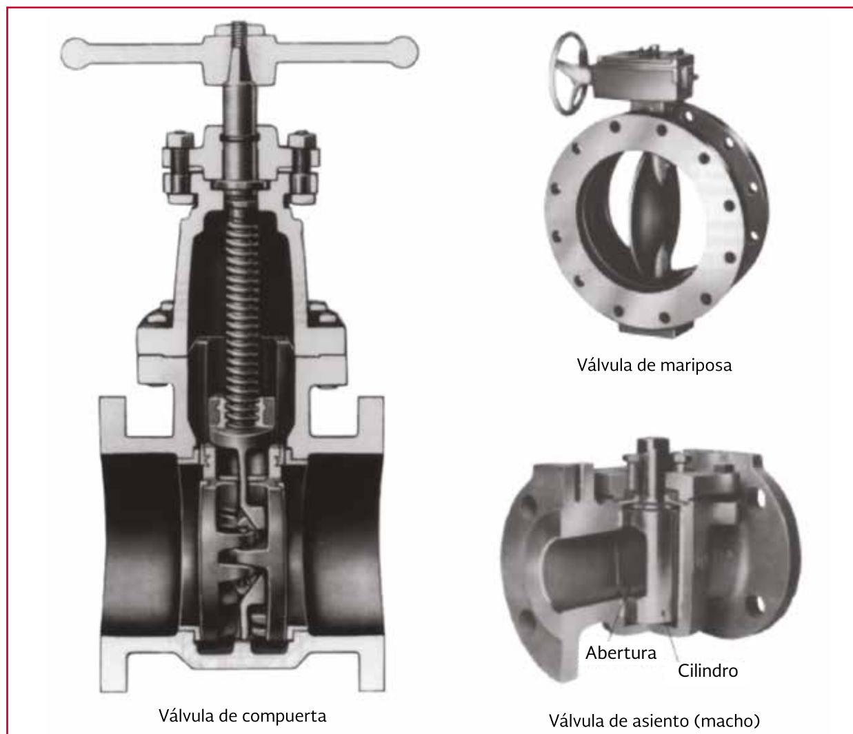
Ilustración 2.12 Válvulas de cierre
