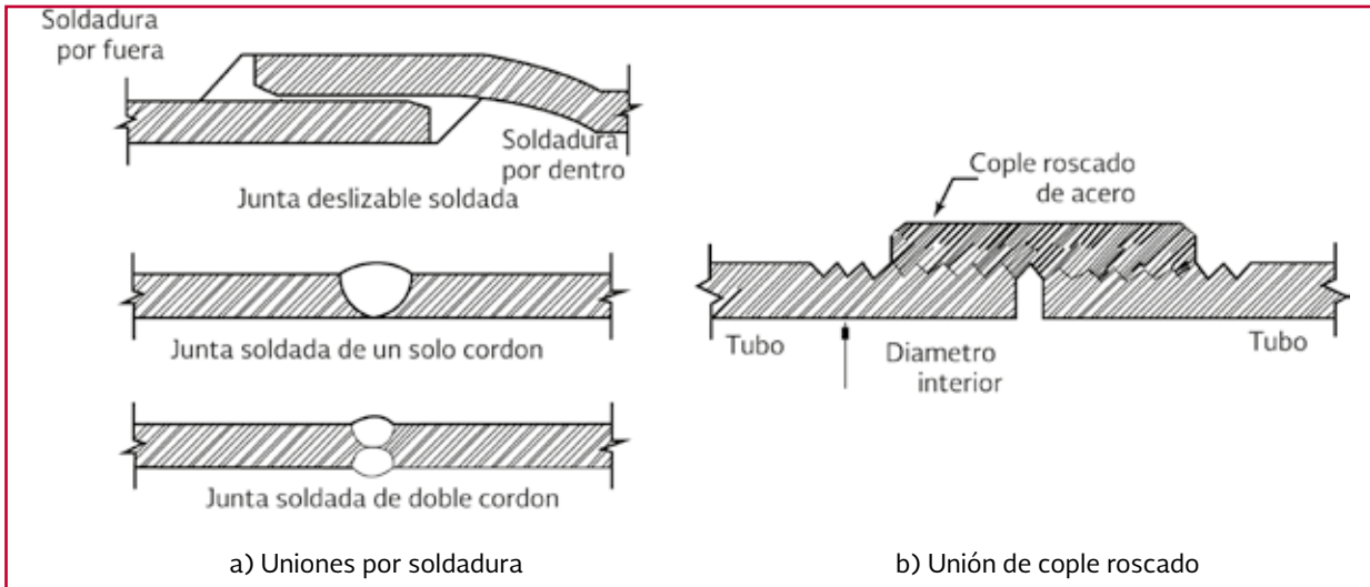
Ilustración 2.9 Uniones para tubería de acero
