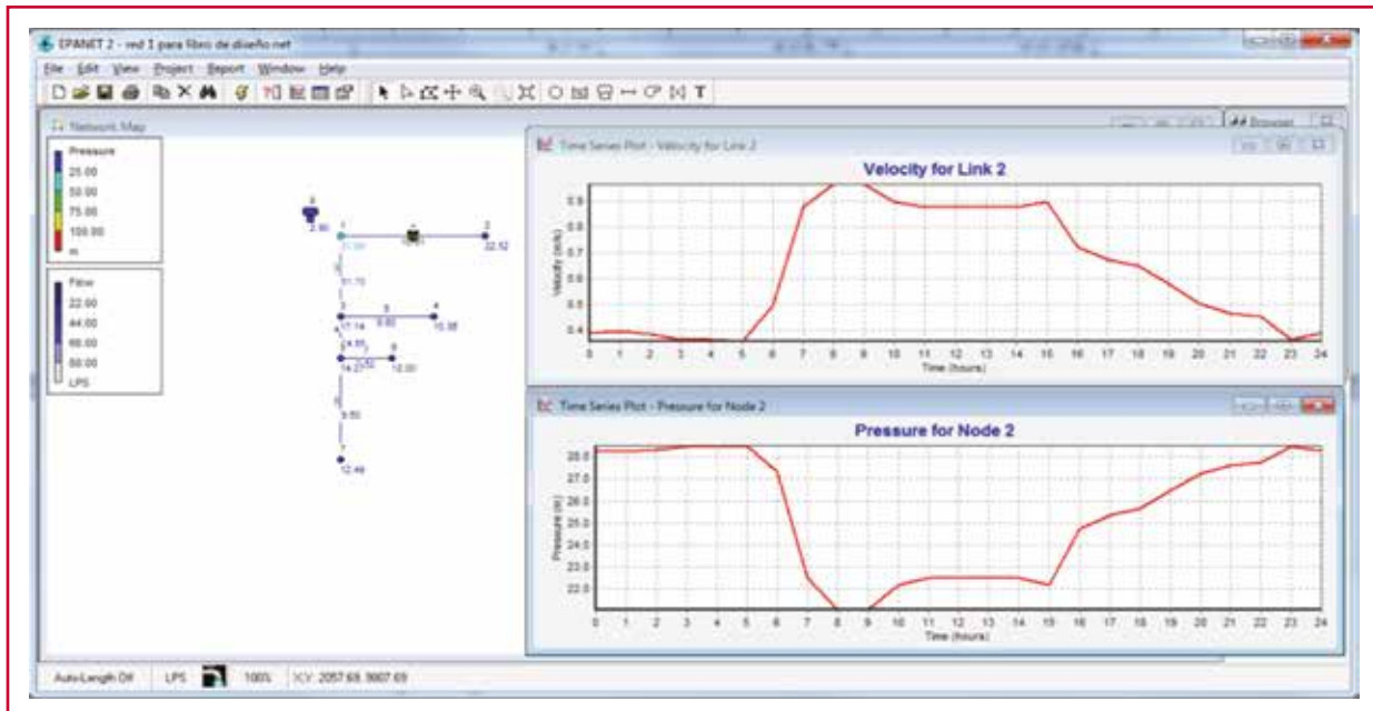
Ilustración 3.18 Velocidad en el tramo 2 y presión en el nodo 2
