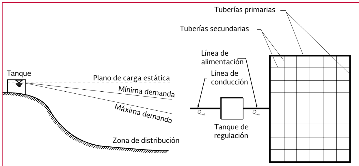
Ilustración 1.6 Distribución por gravedad (recomendable)
