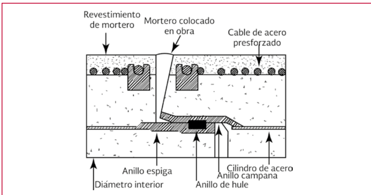
Ilustración 2.8 Unión espiga-campana en tubería de concreto con cilindro de acero
