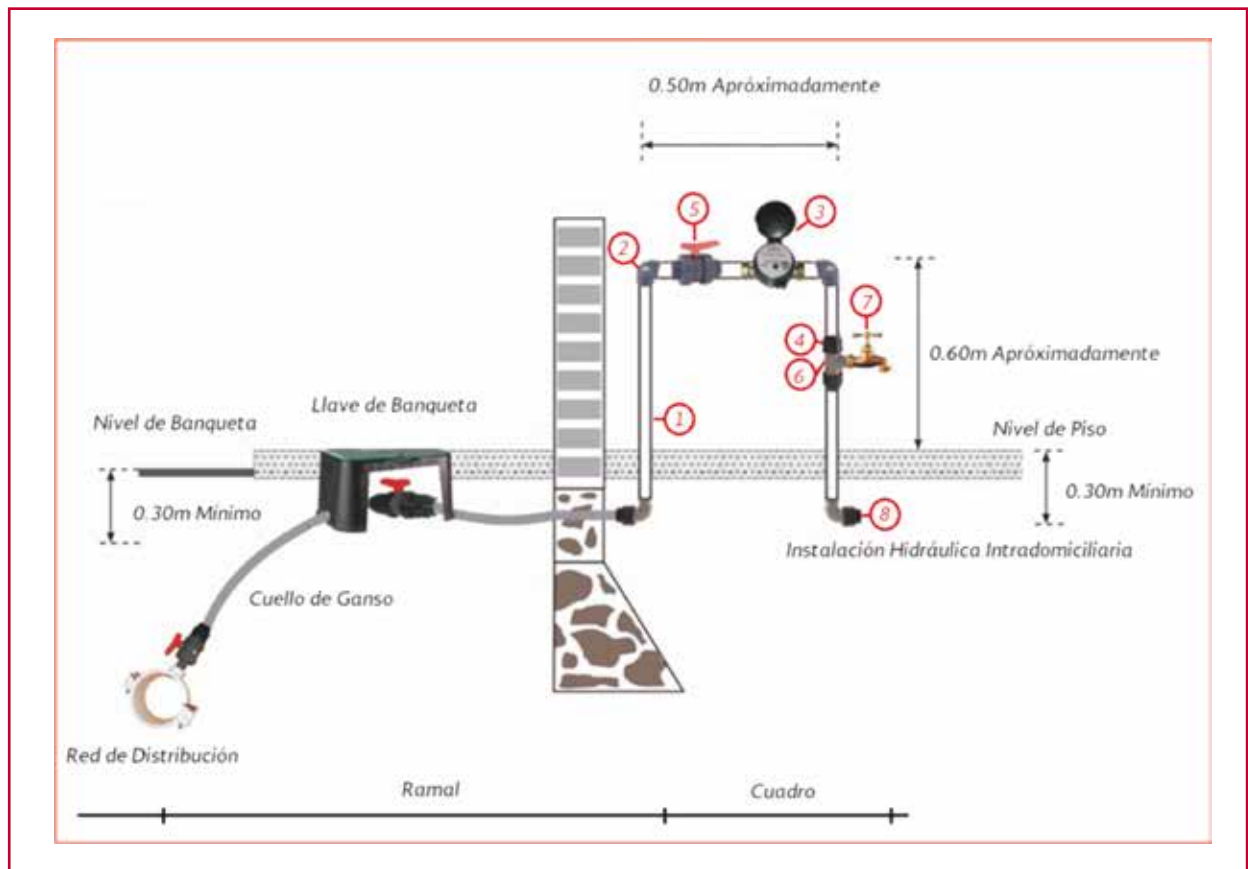
Ilustración 2.44 Toma domiciliaria tipo
