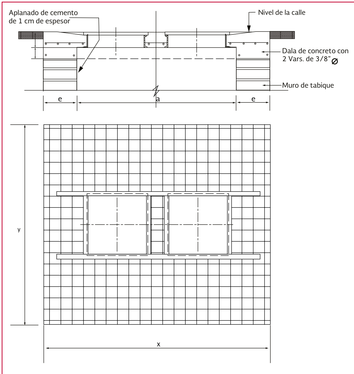
Ilustración 2.28 Caja tipo 6
