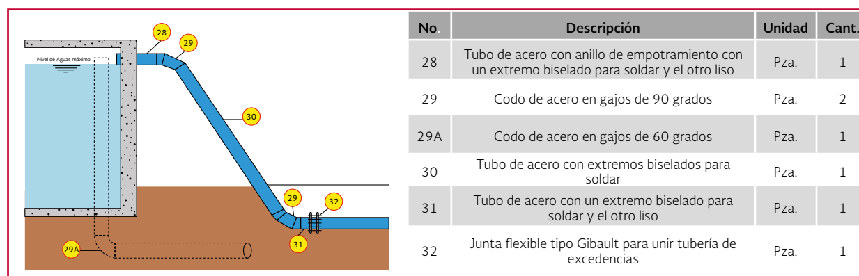
Ilustración 2.40 Fontanería de salida con desagüe de fondo
