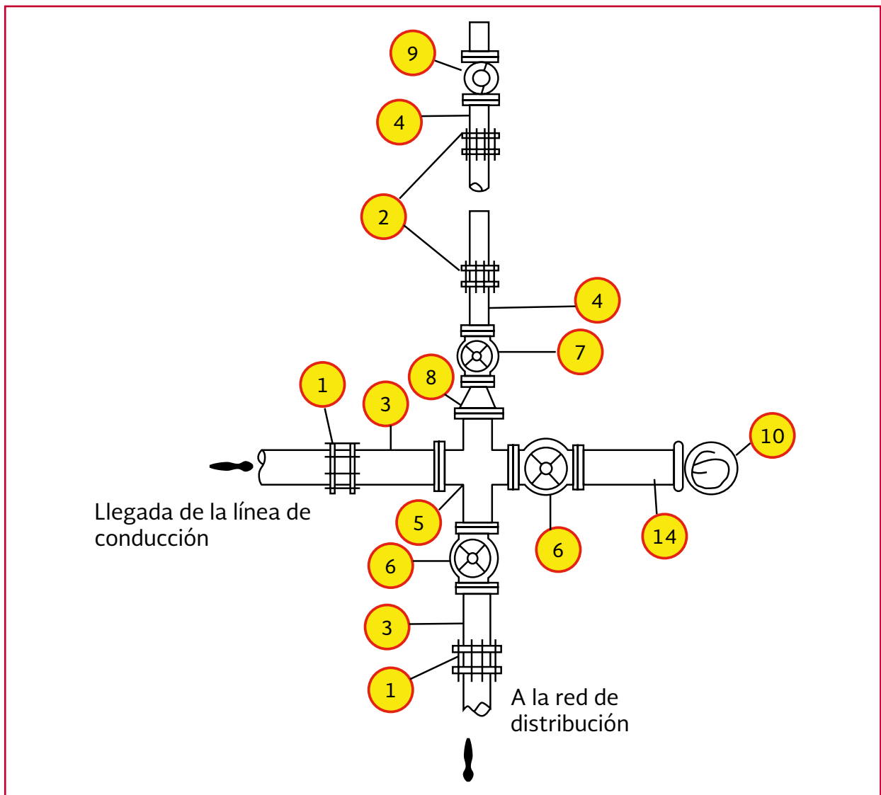
Ilustración 2.42 Tanque elevado, arreglo de fontanería entrada-salida (Planta)
