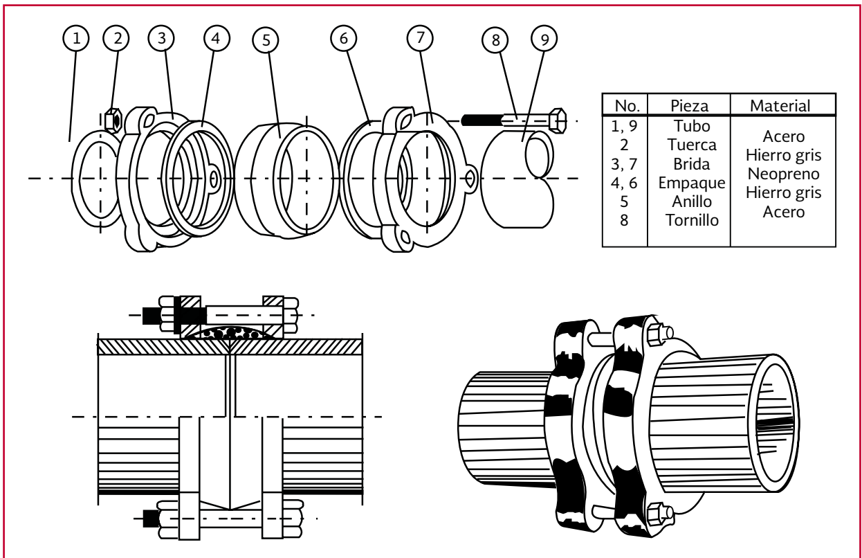
Ilustración 2.4 Junta Gibault
