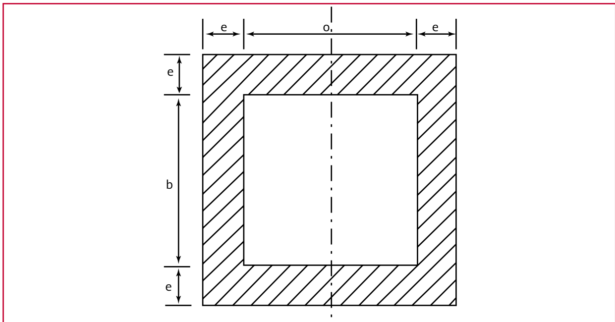
Ilustración 2.20 Caja de operación para válvulas (Planta)
