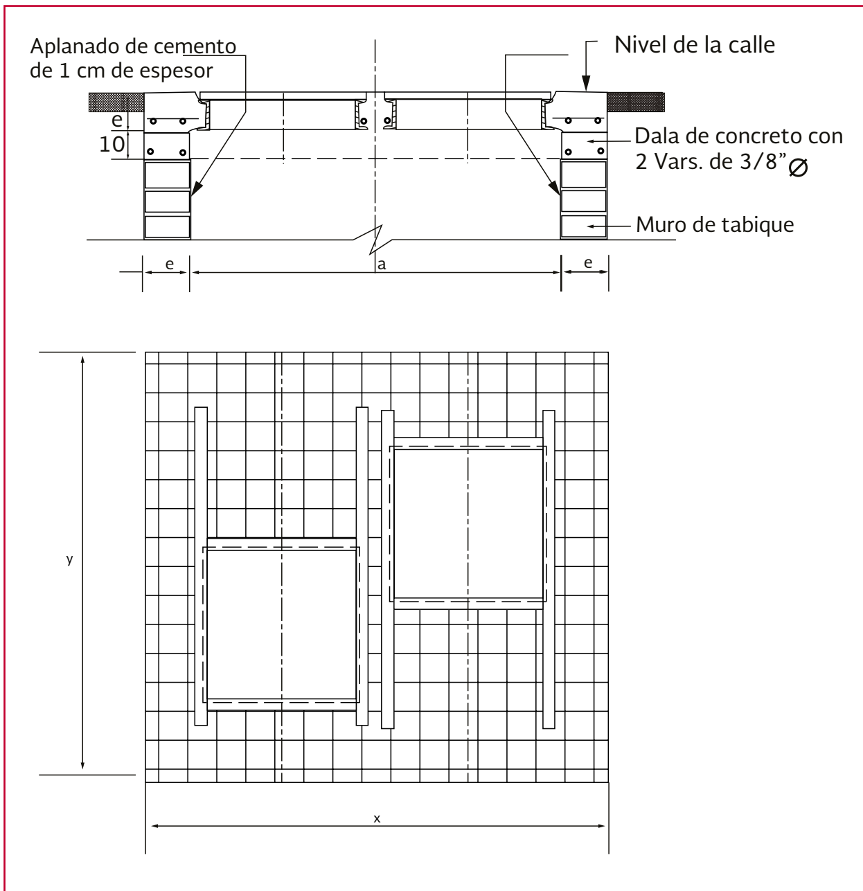
Ilustración 2.32 Caja tipo 10
