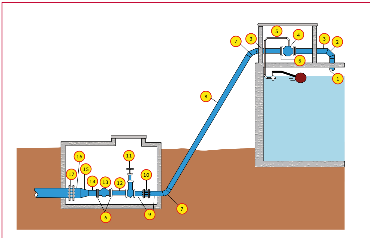
Ilustración 2.37 Tanque superficial. Fontanería de llegada
