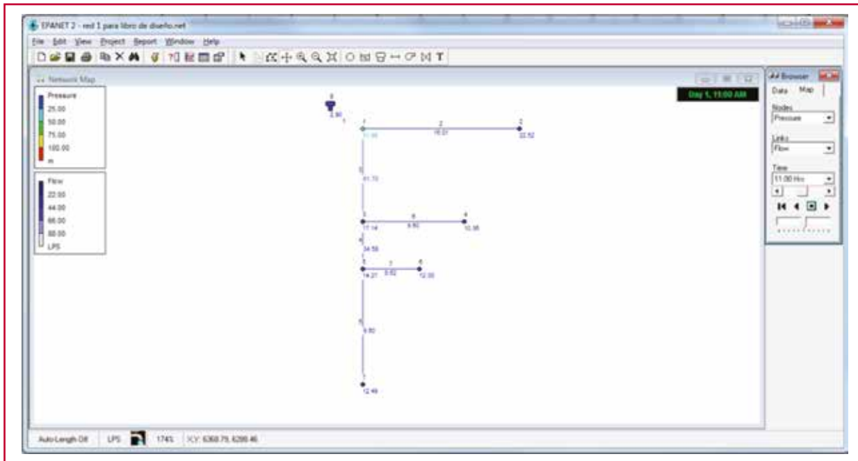
Ilustración 3.16 Resultados de la simulación en los nodos del funcionamiento hidráulico de la red a las 11:00 h
