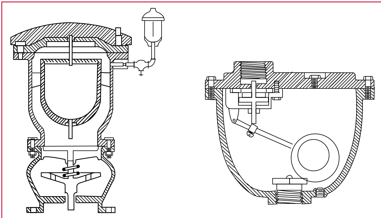
Ilustración 2.14 Válvulas de admisión y expulsión de aire
