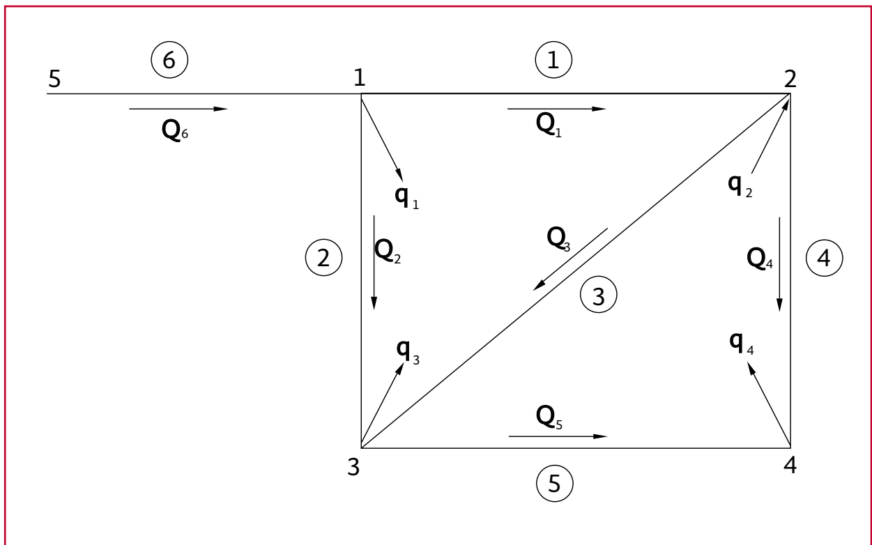
Ilustración 3.3 Red cerrada de tubos
