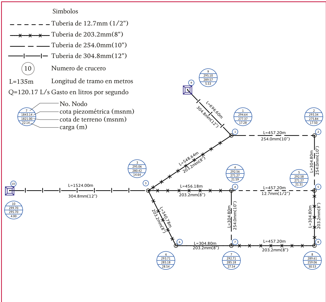
Ilustración 3.7 Resultados para la red del ejemplo 2
