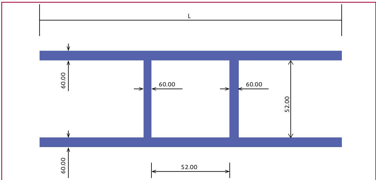
Ilustración 2.22 Dimensiones del contramarco
