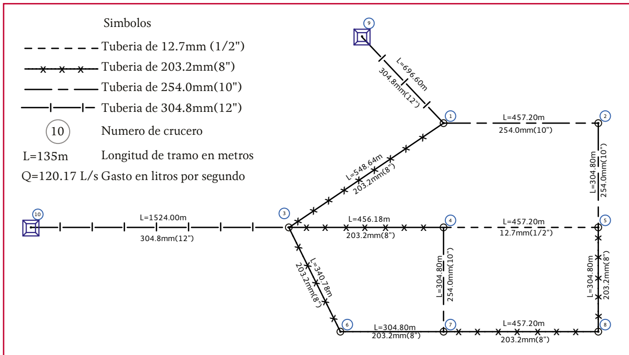
Ilustración 3.6 Red cerrada de distribución de agua potable para ejemplo
