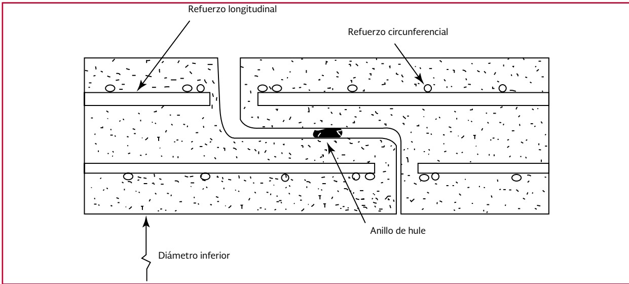
Ilustración 2.7 Unión espiga-campana en tubería de concreto sin cilindro de acero
