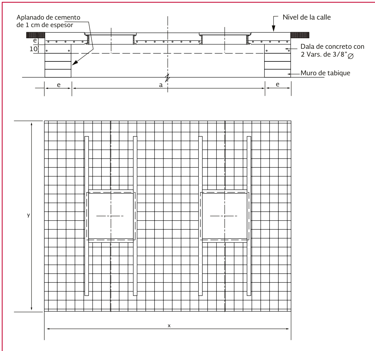
Ilustración 2.30 Caja tipo 8
