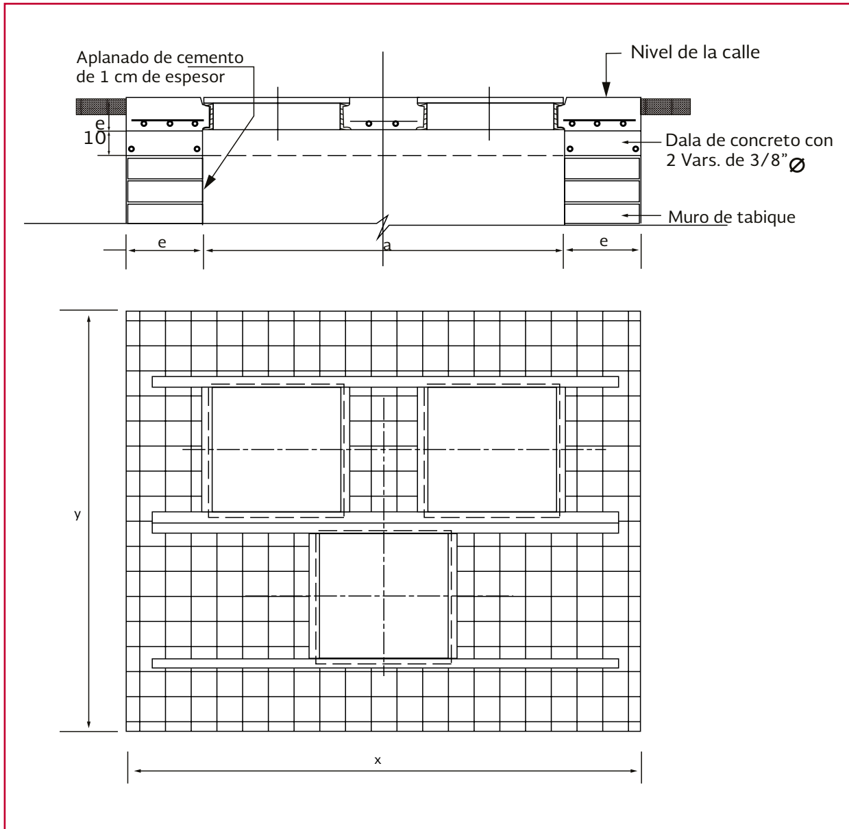
Ilustración 2.34 Caja tipo 12
