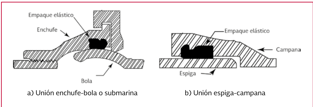
Ilustración 2.6 Uniones para hierro dúctil
