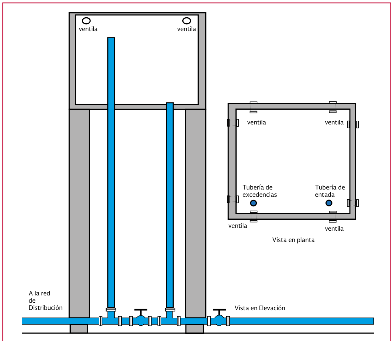
Ilustración 2.41 Tanque elevado, arreglo general de fontanería
