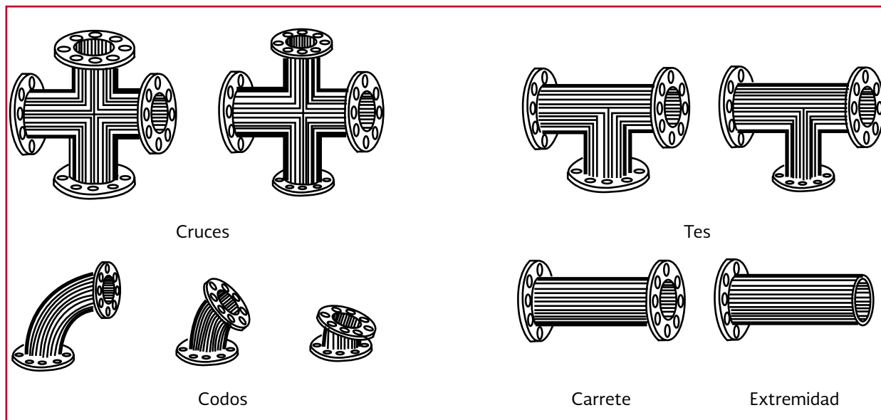
Ilustración 2.11 Piezas especiales de hierro fundido con extremos bridados
