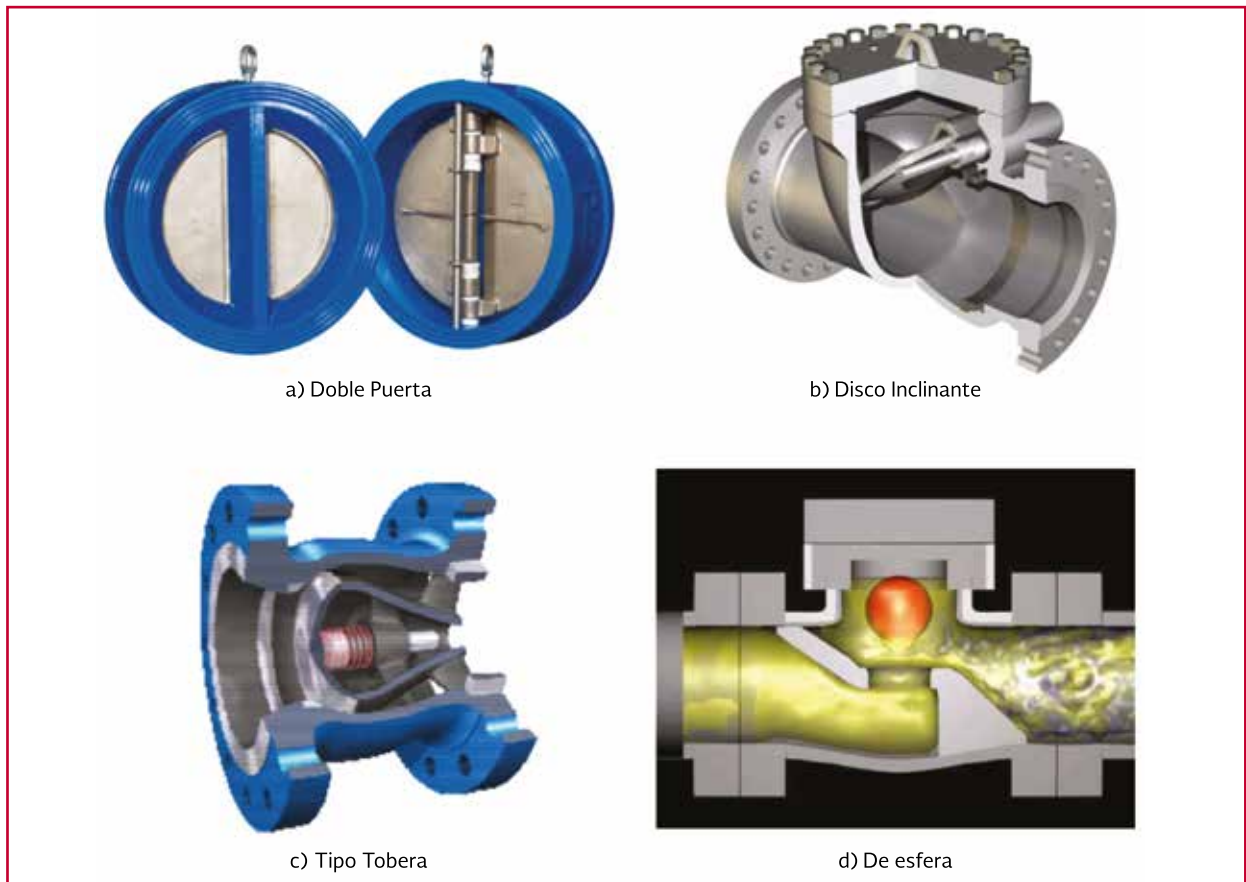
Ilustración 2.16 Válvulas de retención ( check )
