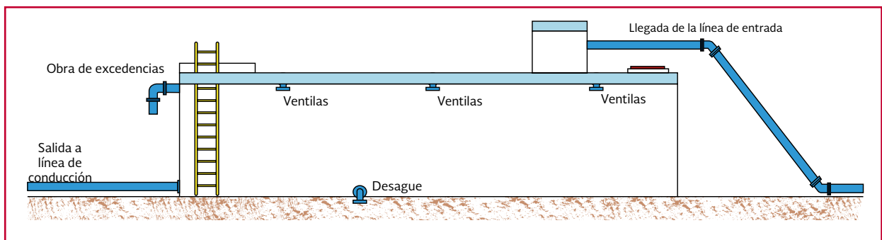
Ilustración 2.36 Tanque superficial, arreglo general de fontanería
