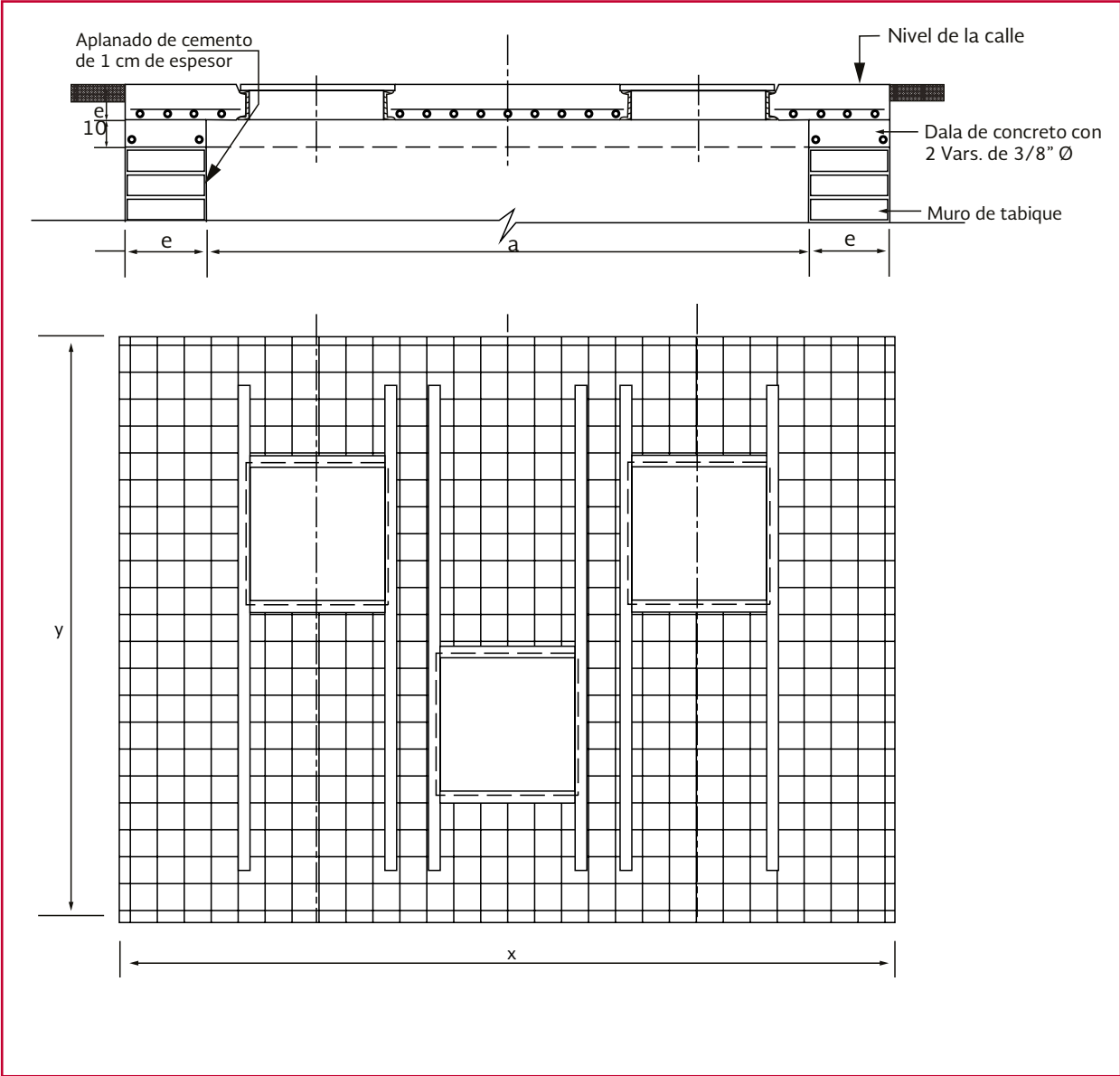
Ilustración 2.35 Caja tipo 13
