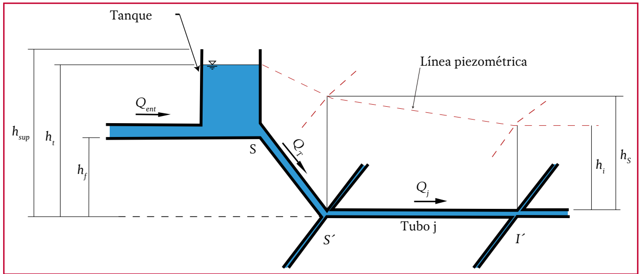
Ilustración 3.12 Consideraciones para las ecuaciones del tanque
