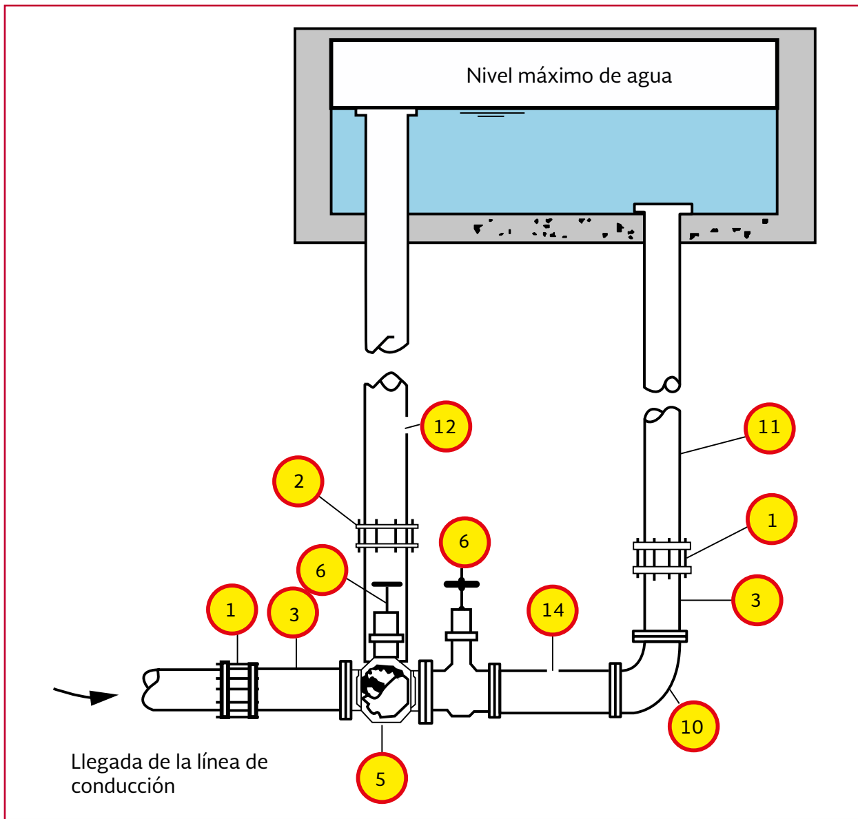
Ilustración 2.43 Tanque elevado, arreglo de fontanería entrada-salida (Elevación)
