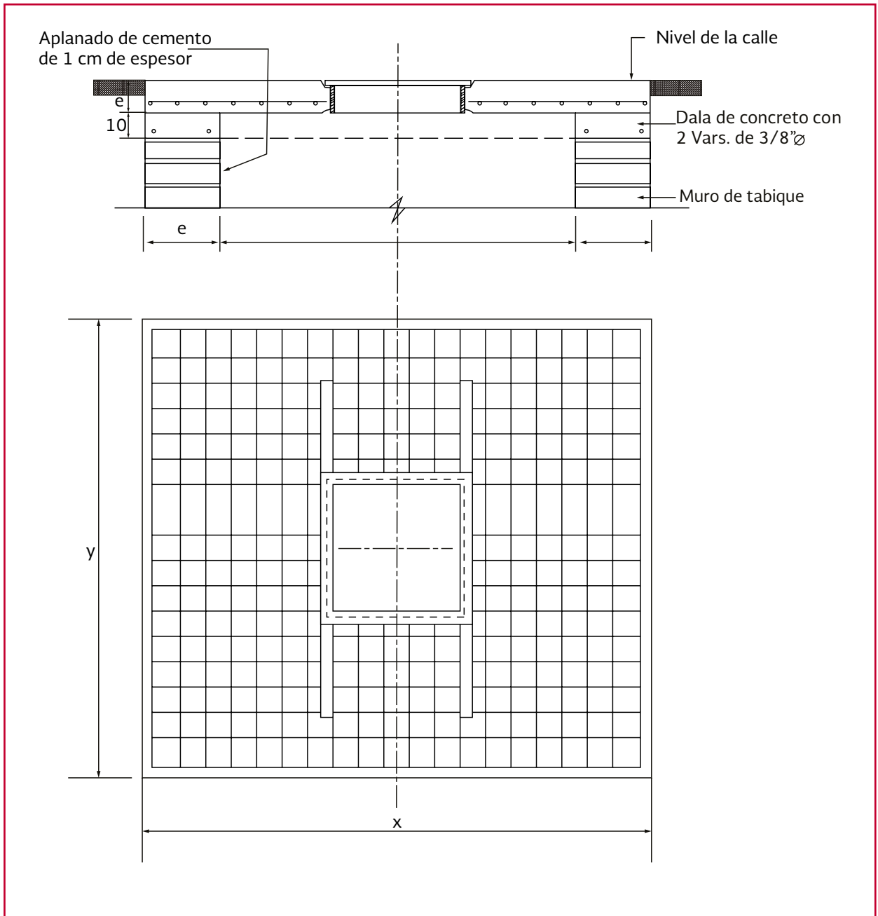
Ilustración 2.25 Caja tipo 3
