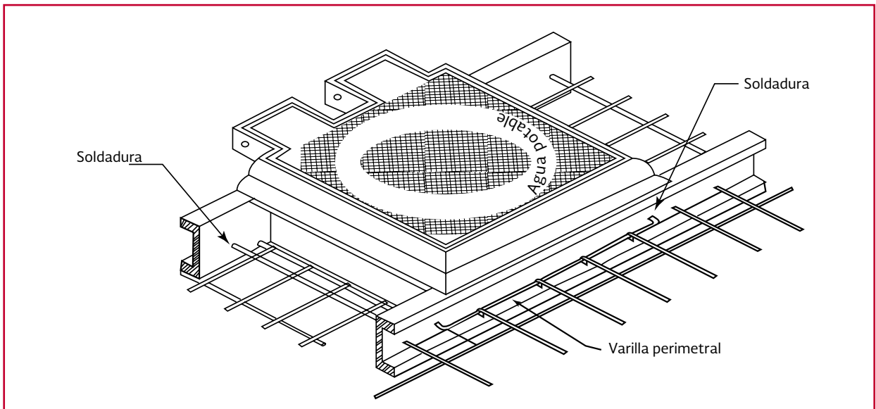
Ilustración 2.21 Armado del contramarco
