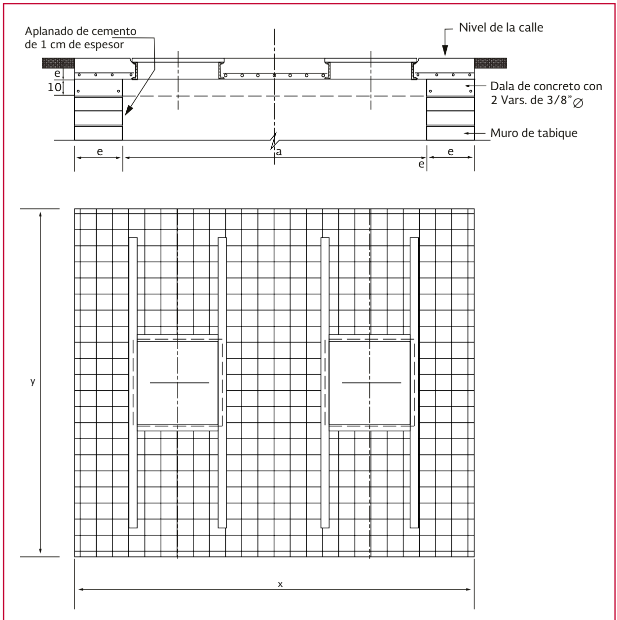
Ilustración 2.29 Caja tipo 7
