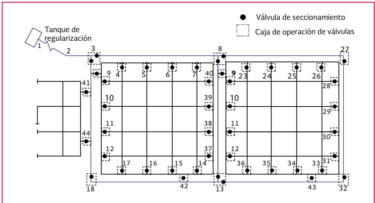
Ilustración 1.4 Red secundaria convencional en bloques
