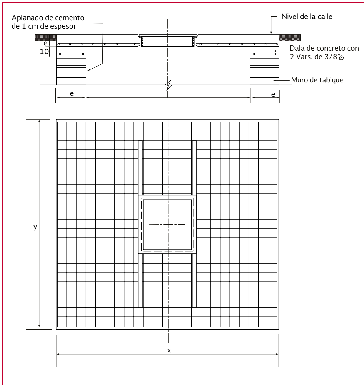
Ilustración 2.26 Caja tipo 4
