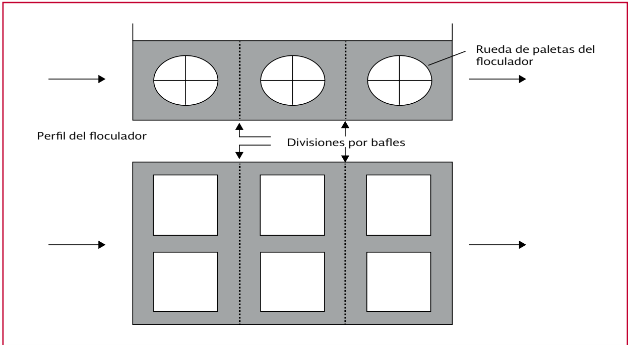
Ilustración 3.25 Detalles del floculador de paletas de rueda
