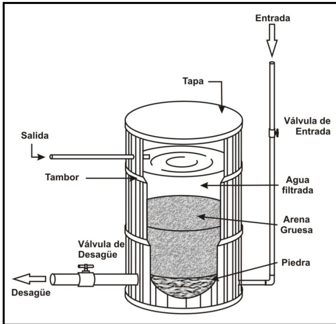
Este es otro diseño de filtro lento no convencional. Aquí, el agua entra por abajo del tambor de 55 galones y fluye hacia arriba a través de la arena
