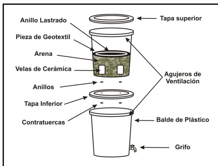
Filtro con velas filtrantes de cerámica y prefiltro de arena
